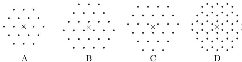
図 9: A, B, C: 立方格子の切断面の x + y + z = 0 への射影。× は原点。 A は x + y + z = 0 、B は x + y + z = 1 、C は x + y + z = 2 。D: C と D を合わせたもの。
