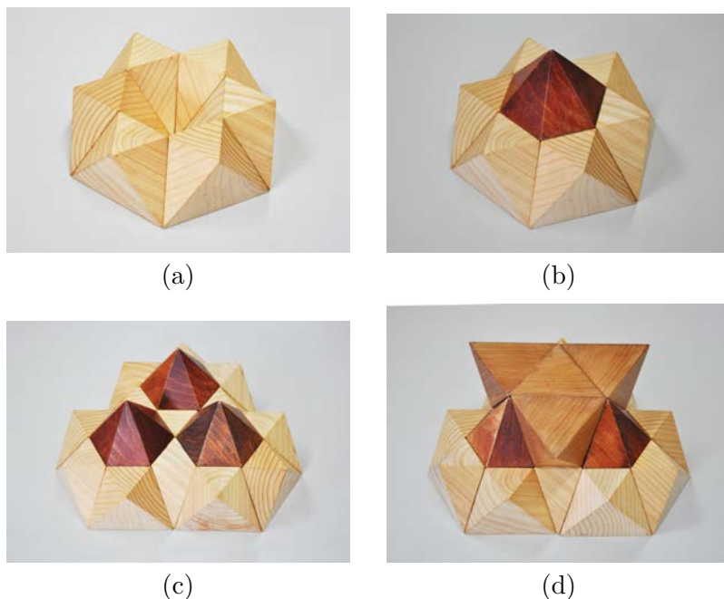
図 4: H と T による 3 次元空間充填
